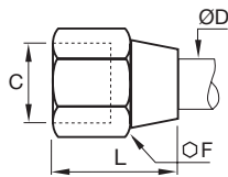
Écrou 0110..60
