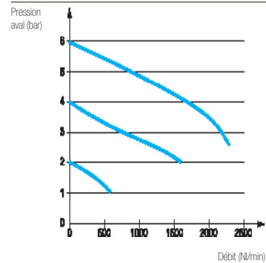
Modèles G3/8
